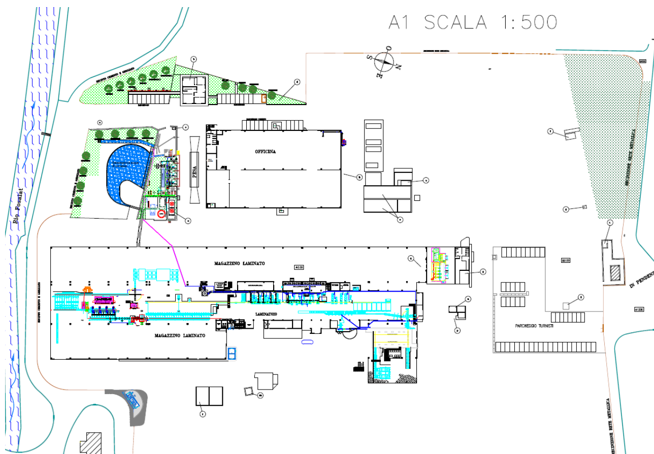
Figura 3.3.2 - Planimetria del sito Acciaierie Venete S.p.A. di Buja
